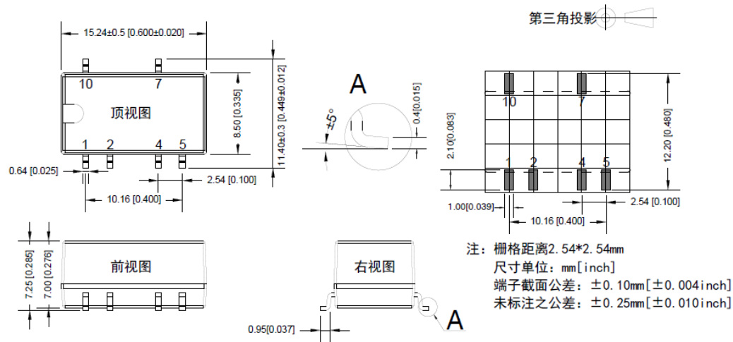
封装尺寸图
