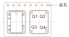
Pin1在料带上的象限位置
